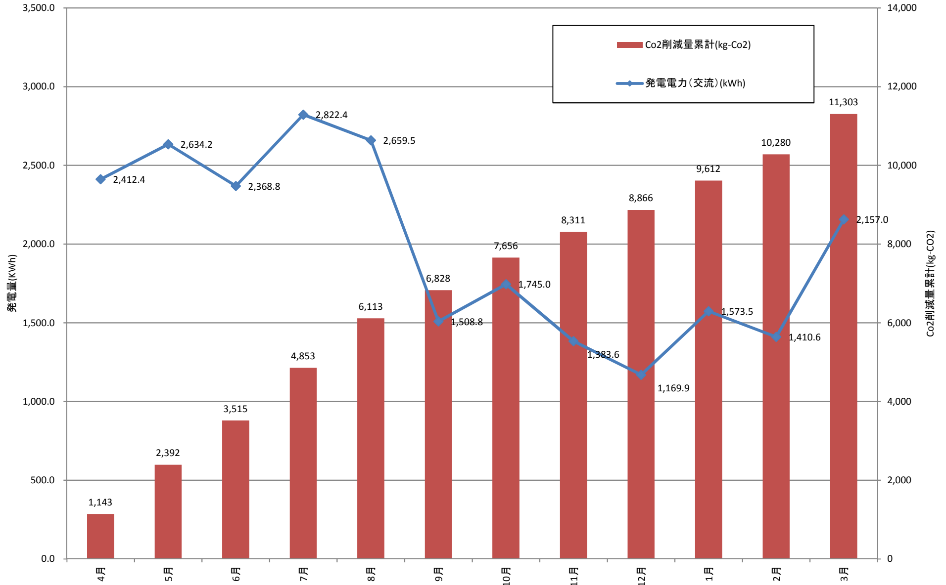
平成30年度 太陽光発電状況
