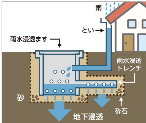
雨水浸透ます・雨水浸透トレンチ
