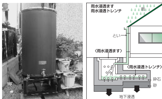
雨水貯留槽
