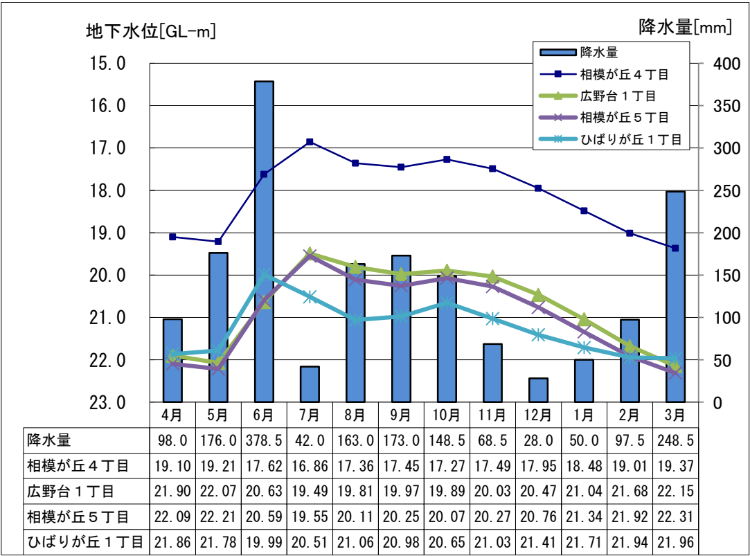
令和5年度 降水量と月平均地下水位(台地部)(図4-3)
