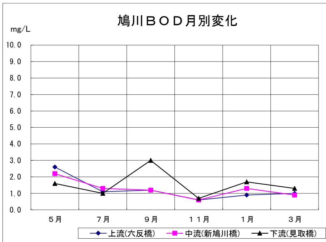
令和5年度 鳩川BOD月別変化(図2-2-1)
