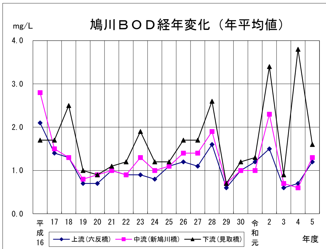
令和5年度 鳩川BOD経年変化(図2-2-2)
