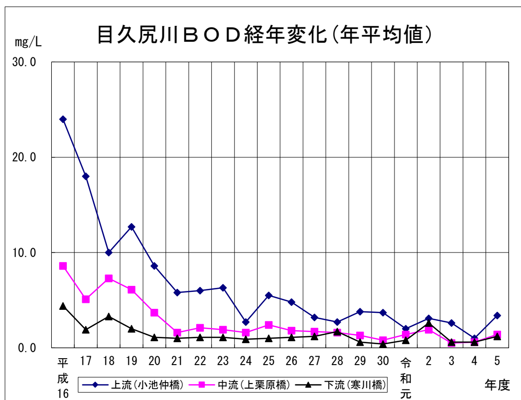
令和5年度 目久尻川BOD経年変化(図2-3-2)
