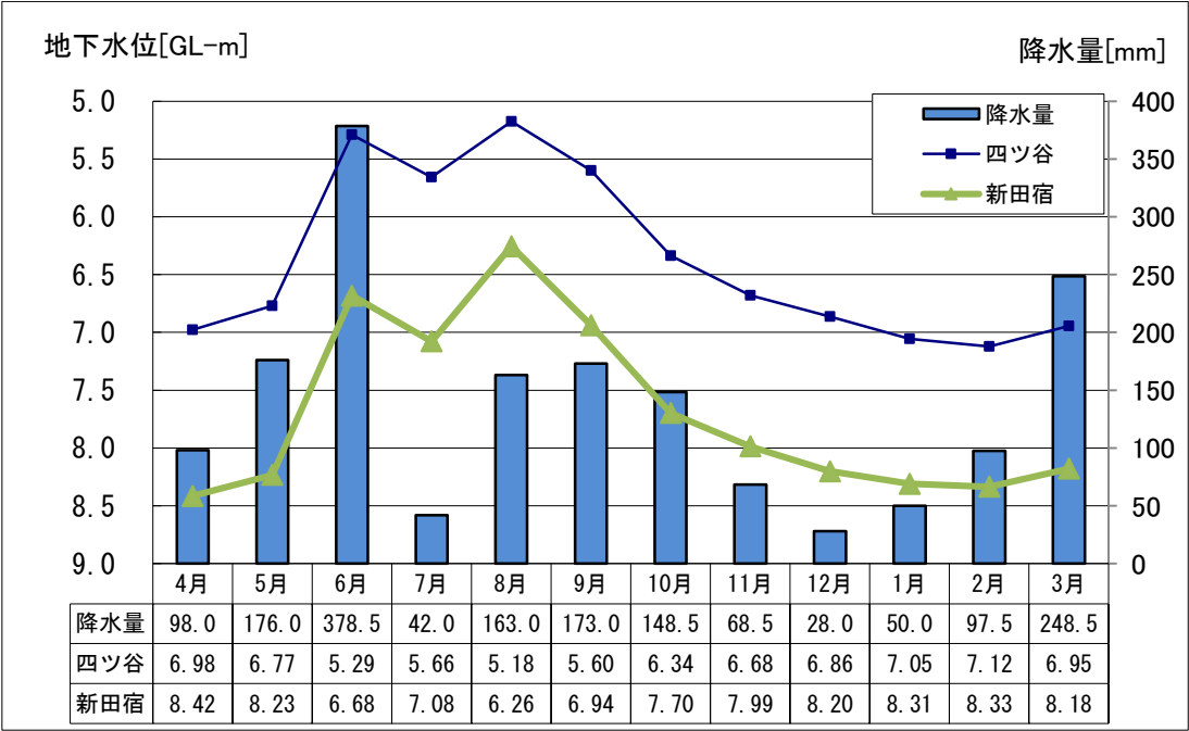
令和5年度 降水量と月平均地下水位(台地部)(図4-3)
