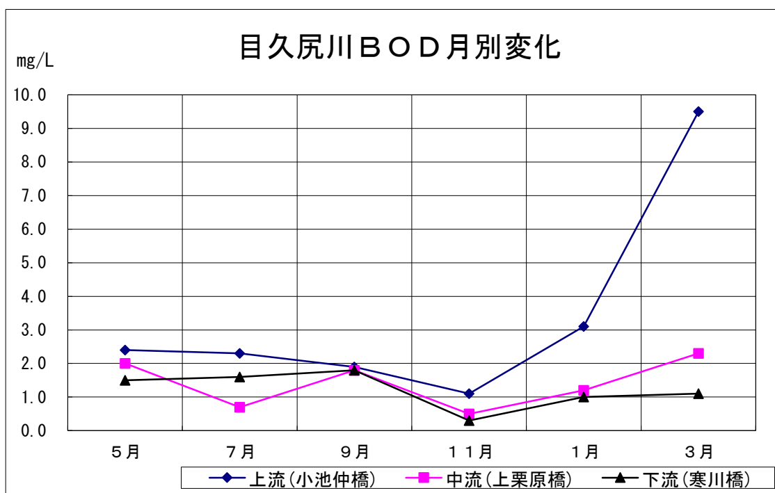
令和5年度 目久尻川BOD月別変化(図2-3-1)
