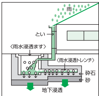
雨水浸透ます・トレンチ
