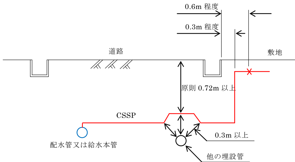
道路内横断配管例（口径 50mm 以下）
