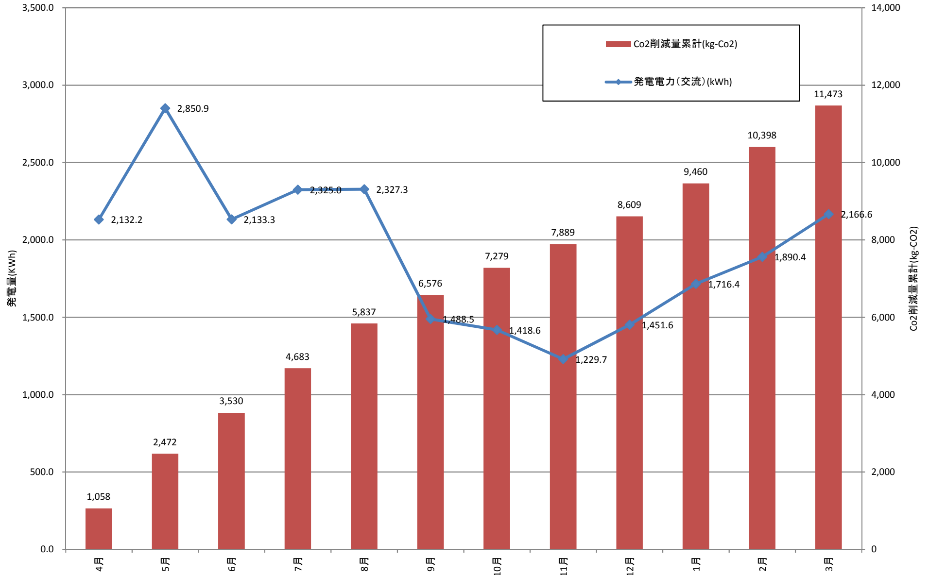
平成28年度 太陽光発電状況
