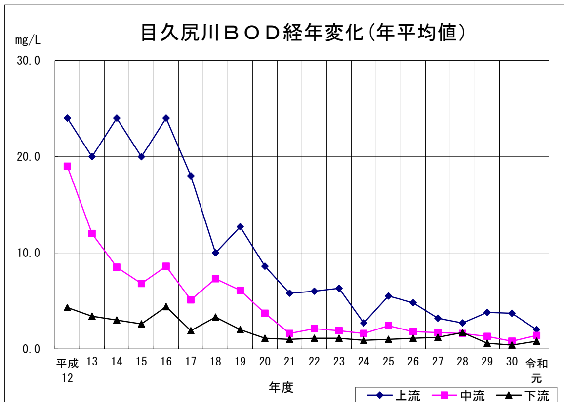
令和元年度 目久尻川BOD経年変化(図3-3-2)
