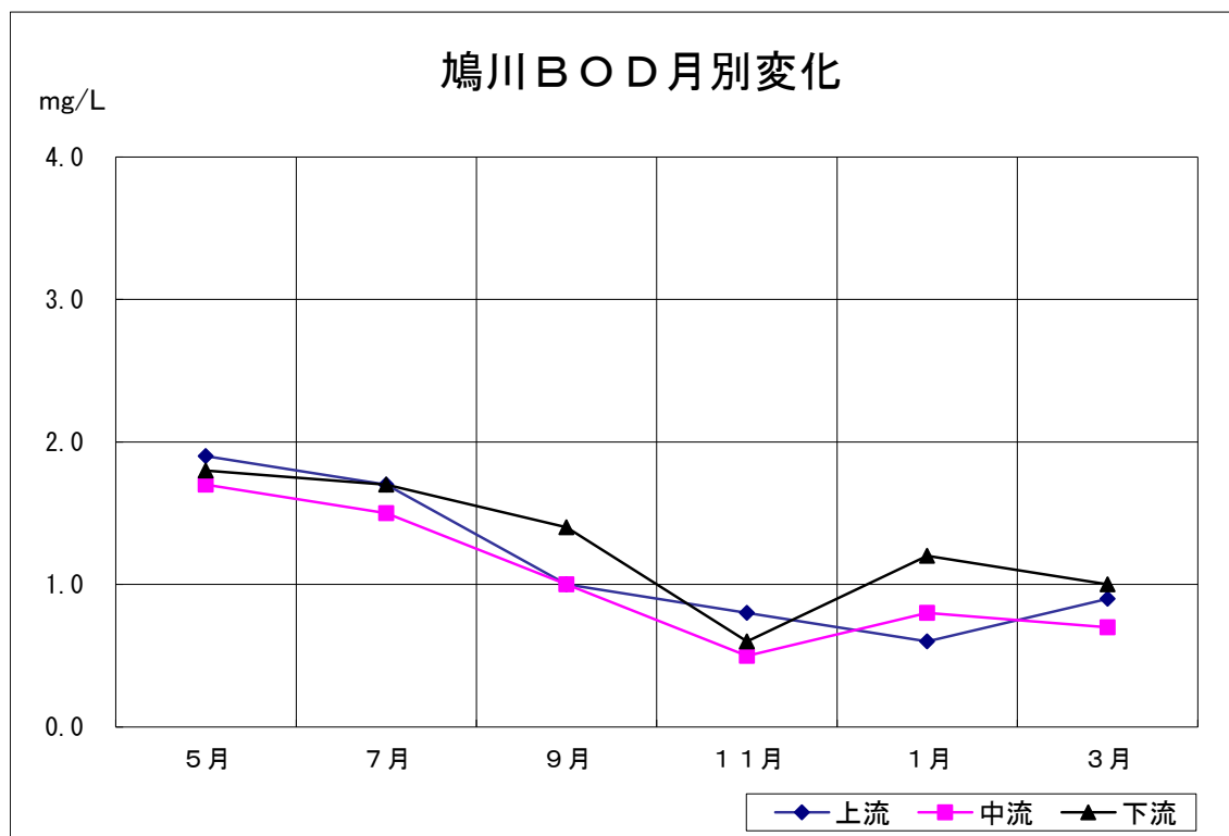
令和元年度 鳩川BOD月別変化(図3-2-1)
