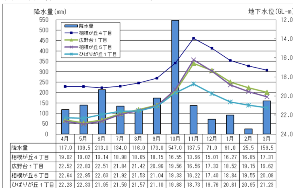
令和元年度 降水量と月平均地下水位(台地部)(図5-3)
