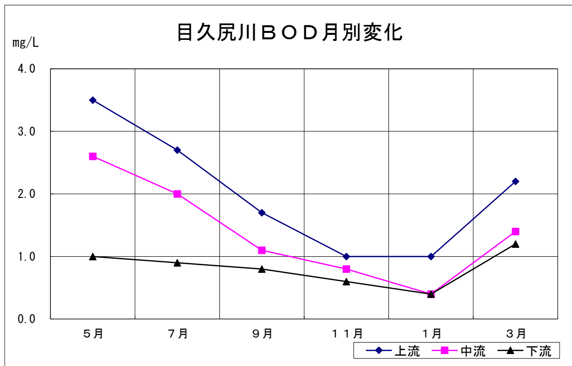
令和元年度 目久尻川BOD月別変化(図3-3-1)
