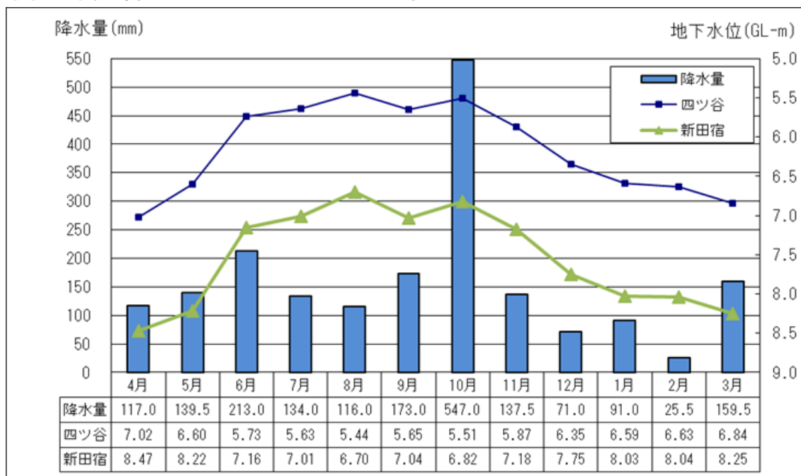
令和元年度 降水量と月平均地下水位(低地部)(図5-2)
