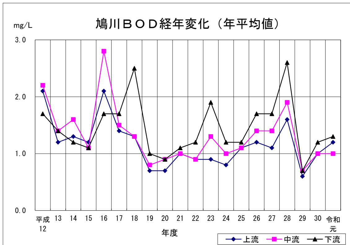
令和元年度 鳩川BOD経年変化(図3-2-2)
